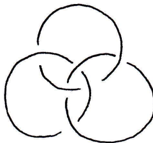
ボロミアンリング
