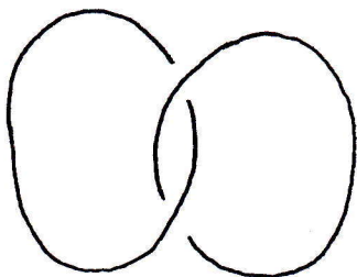
ホップ絡み目
