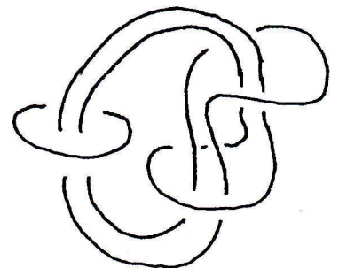
リボン絡み目
