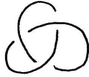
3葉結び目 K_{31}
