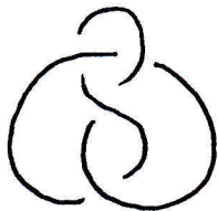
8の字結び目 K_{41}
