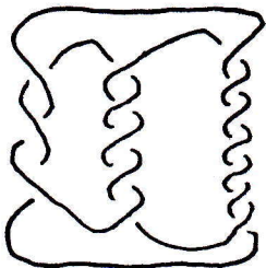
(-3,5,7) フレツェル結び目
