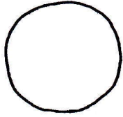
自明な結び目 K_0
